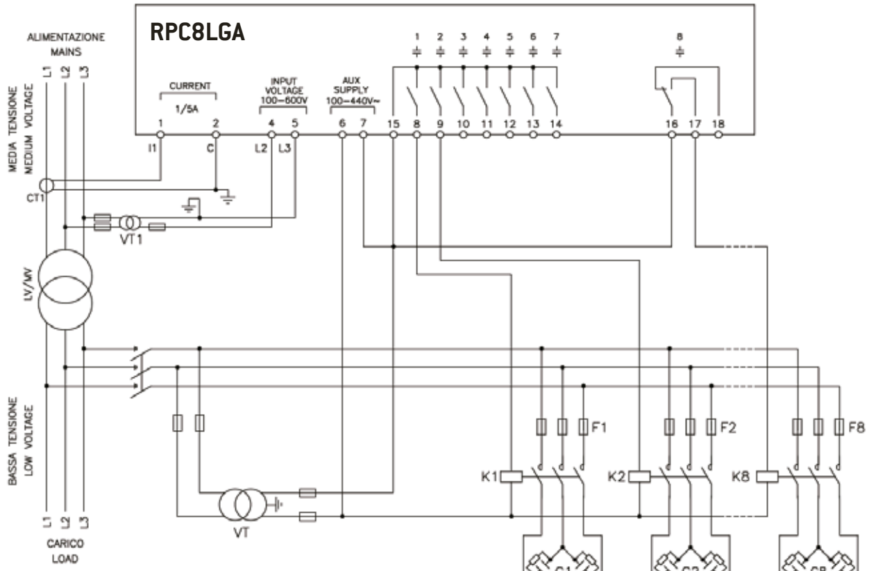
Conexión con medida y corrección del factor de potencia en MT
